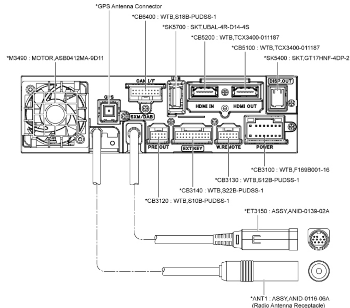
*ET3150 : ASSY,ANID-0139-02A
