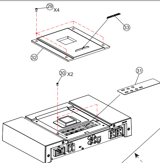
PL00037A 4CH MAIN-P.W.Board
