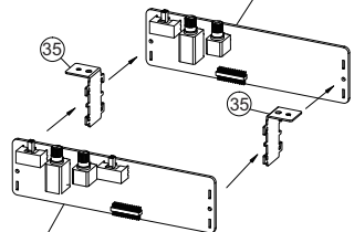
PL00037A SUB2-P.W.Board
